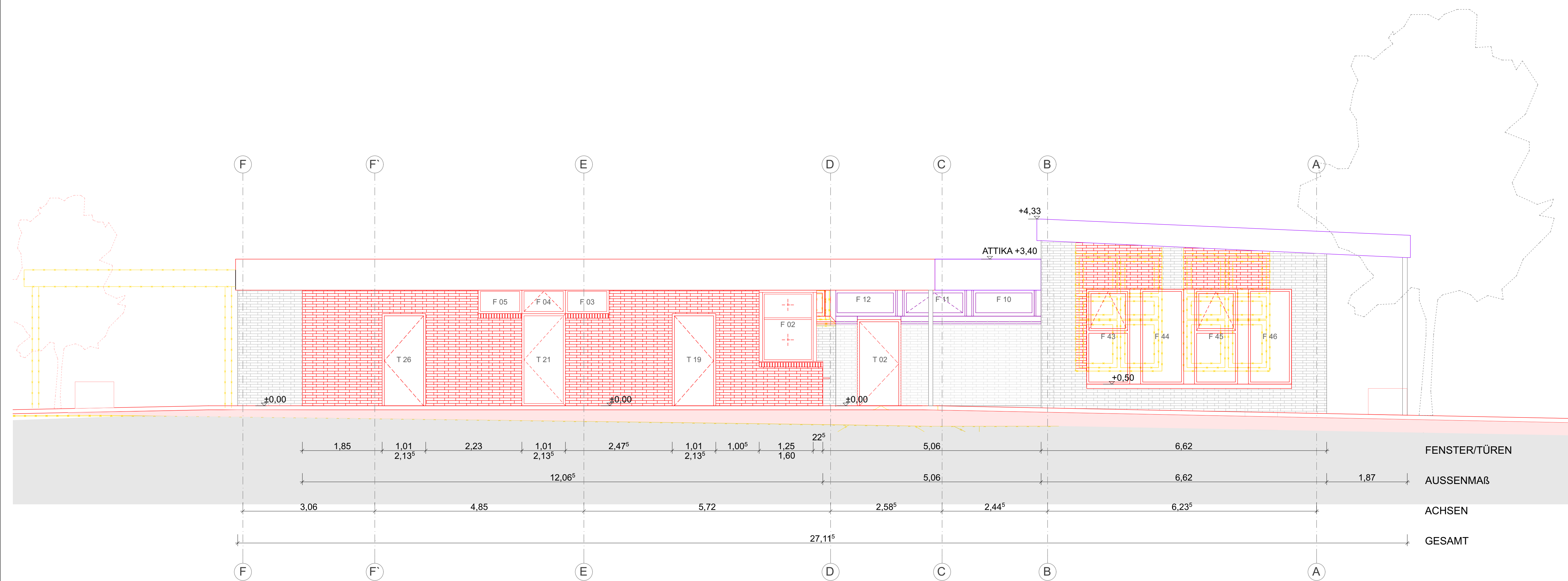
ANSICHT SW 1:50
