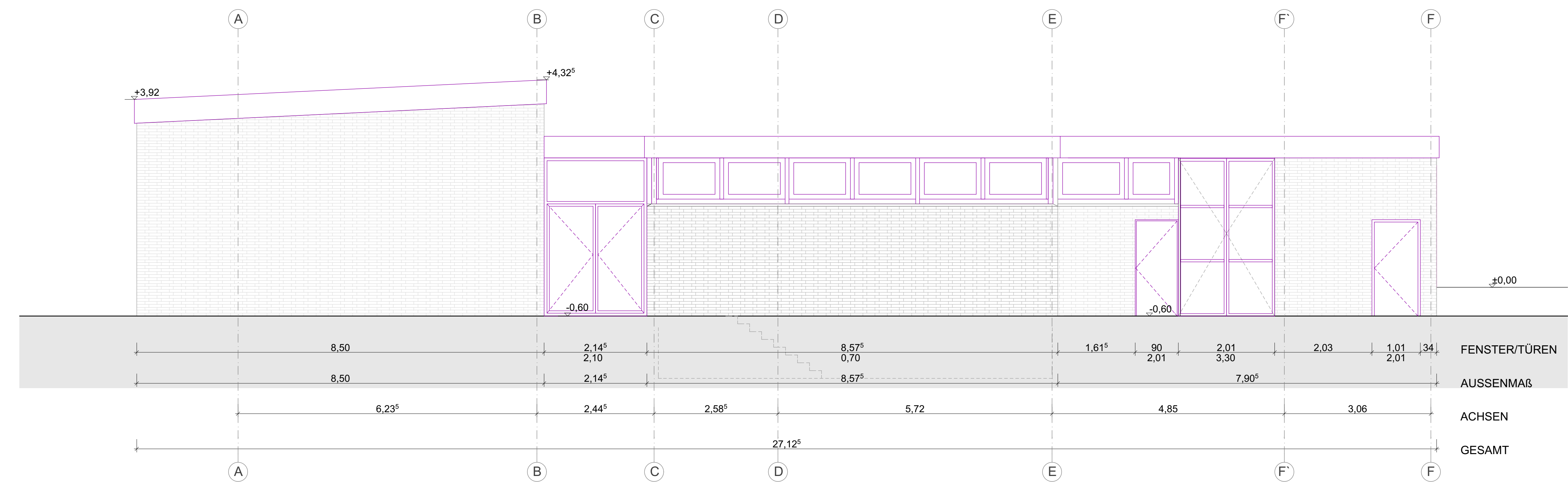
ANSICHT NO 1:50
