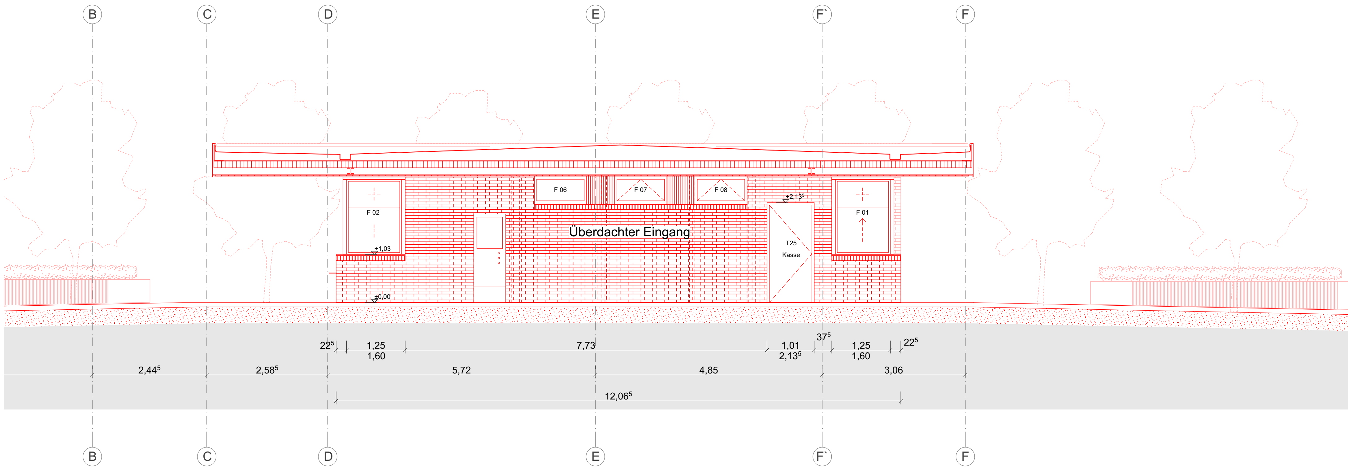
SNITT E-E 1:50
