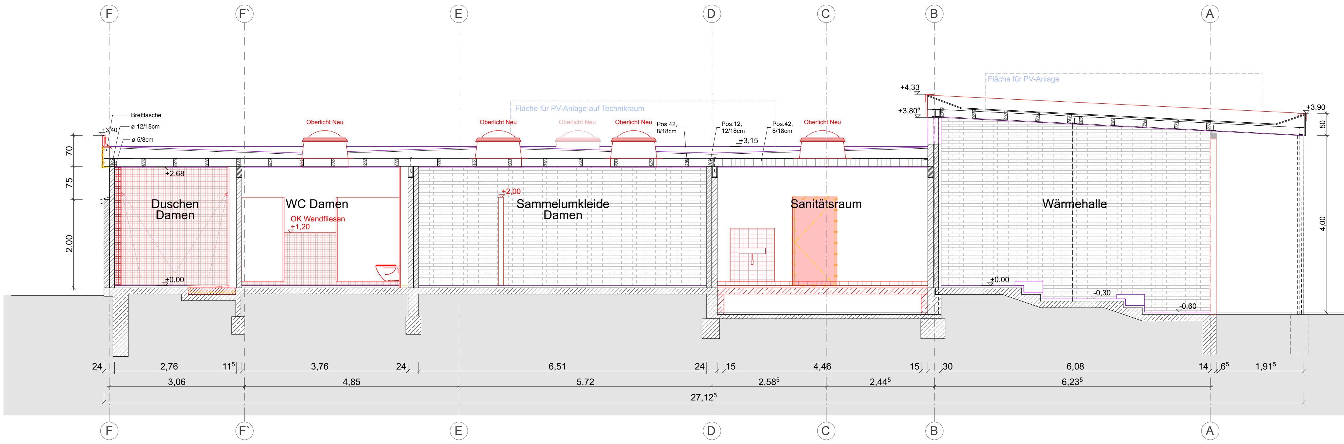
SNITT A-A 1:50
